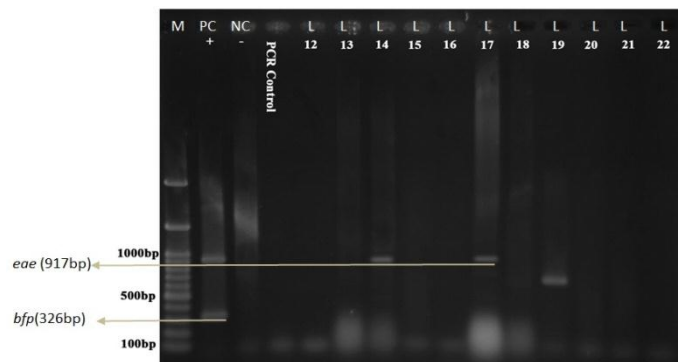
شکل شماره ۱. محصول PCR بر روی ژل مربوط به ژن eae و bfp ، به ترتیب از چپ به راست، کنترل مثبت (PC)، کنترل منفی (NC)، نمونه های ۱۲-۲۲ نمونه های E.coli بالینی جدا شده از نمونه های اسهالی، نمونه ۱۴ و ۱۷ دارای ژن eae با طول ۹۱۷ می باشند.
