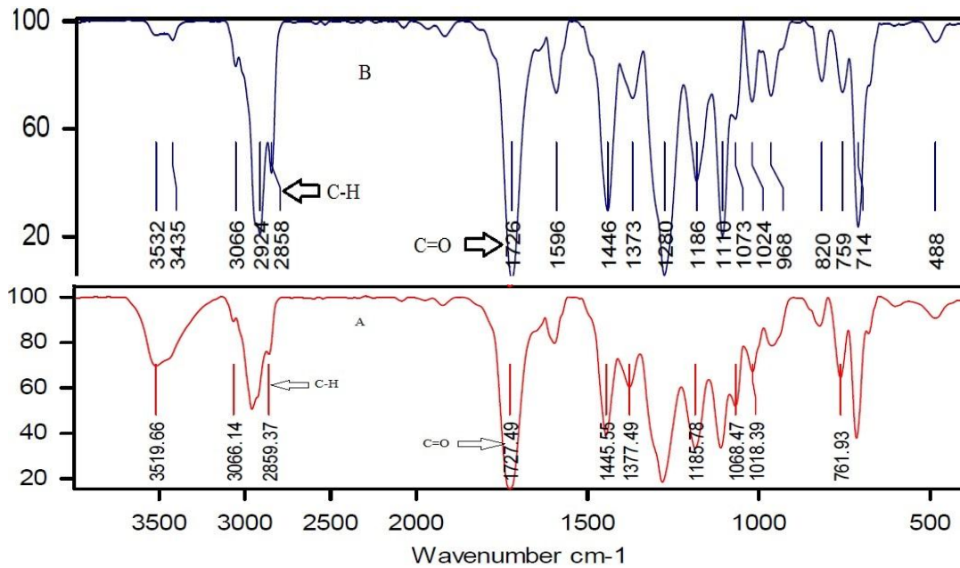
شکل ۴. نمودار A، FTIR مربوط به PHB استاندارد و B، FTIR مربوط به PHB تولید شده توسط باسیلوس
