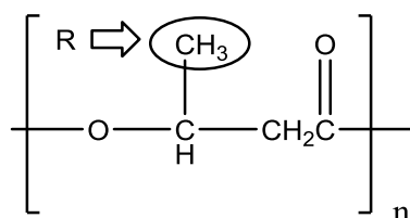
شکل ۱. ساختار و گروه جانبی پلی هیدروکسی بوتیرات (۱۲).
