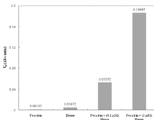
شکل شماره ۴. سرعت اکسیداسیون TMB توسط فریتین به تنهایی، هیم به تنهایی و نیز فریتین در حضور غلظت های ۰/۱ و ۱ میکرو مولار هیم.
