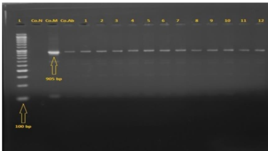
شکل شماره ۵. نتایج PCR ژن ۱۶SrRNA باکتری بروسلا روی ژل آگارز ۱ درصد. ستون L. مارکر ۱۰۰bp؛ Co.N. کنترل منفی؛ Co.M. کنترل مثبت بروسلا ملی تنسیس؛ Co.Ab. کنترل مثبت بروسلا آبوروس؛ ستون‌های شماره ۶-۱۱. نمونه‌های گوسفند؛ ۷-۱۱. نمونه‌های بز و شماره ۱۲. نمونه انسانی از شهرستان هلیلان
