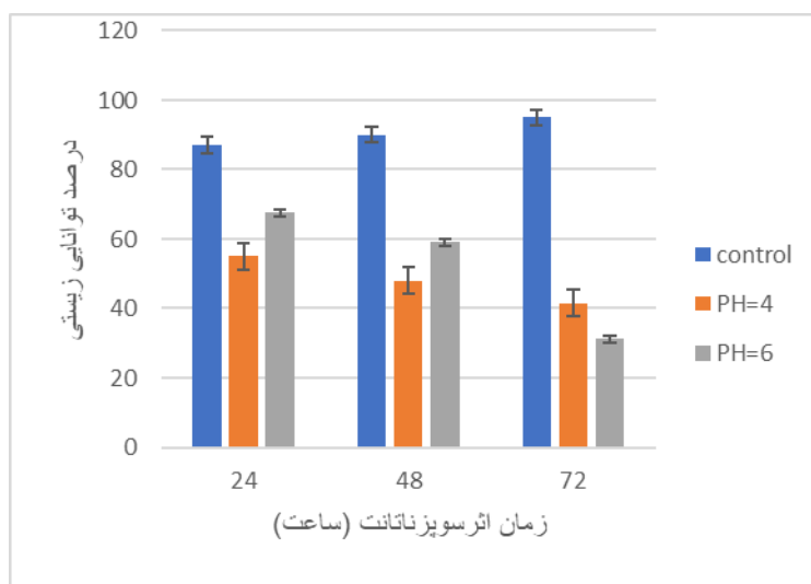
نمودار شماره ۱. مقایسه درصد زنده‌مانی پروبیوتیک بیفیدوباکتریوم بر رده سلول سرطانی AGS
