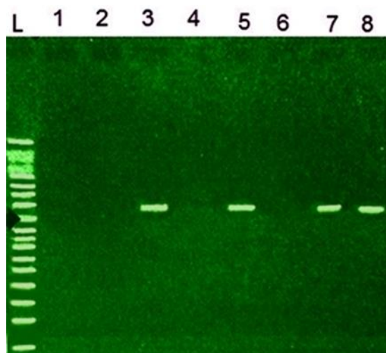
شکل شماره ۱. اندازه مولکولی محصول Gly56Ala PCR تکثیرشده در افراد بیمار و سالم (کنترل) برای آلل چندشکلی؛ DNA Ladder: Allele:- (521 bp) و 50 bp
