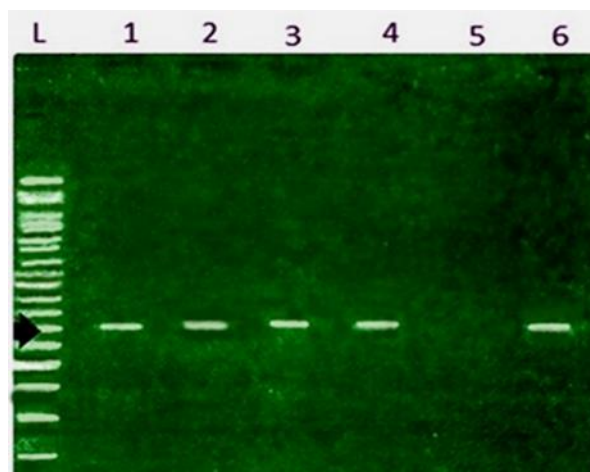
شکل شماره ۲. اندازه مولکولی محصول Gly56Ala PCR تکثیرشده در افراد بیمار و سالم (کنترل)؛ DNA Ladder: 50 bp و Allele:G (300 bp)
