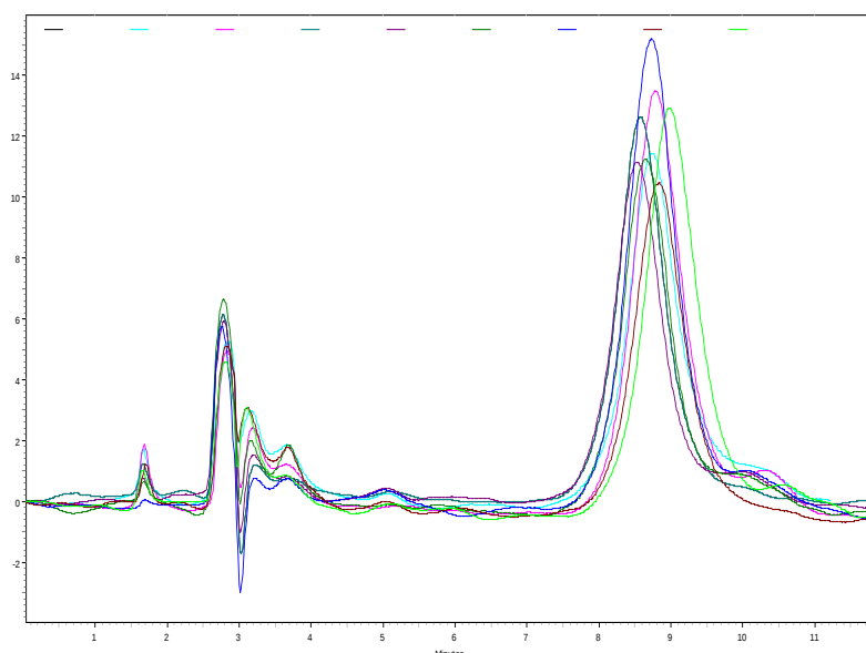
شکل شماره ۳. روماتوگرام‌های HPLC مربوط به ارگوسترول استخراج شده از سلول‌های کاندیدا/گلابراتای تحت تیمار با غلظت‌های مختلف آنتول.
