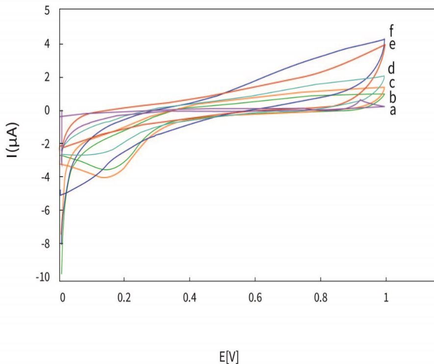
شکل شماره ۳. ولتاموگرام‌های ثبت شده از زیست حسگر مبتنی بر گلوتامات اکسیداز در غلظت‌های مختلف گلوتامات، غلظت (a) ۶۳ μM، (b) ۱۲۵ μM، (c) ۲۵۰ μM، (d) ۵۰۰ μM، (e) ۷۵۰ μM، (f) ۱ mM، دما ۲۵ درجه سانتی‌گراد و pH ۷/۴
