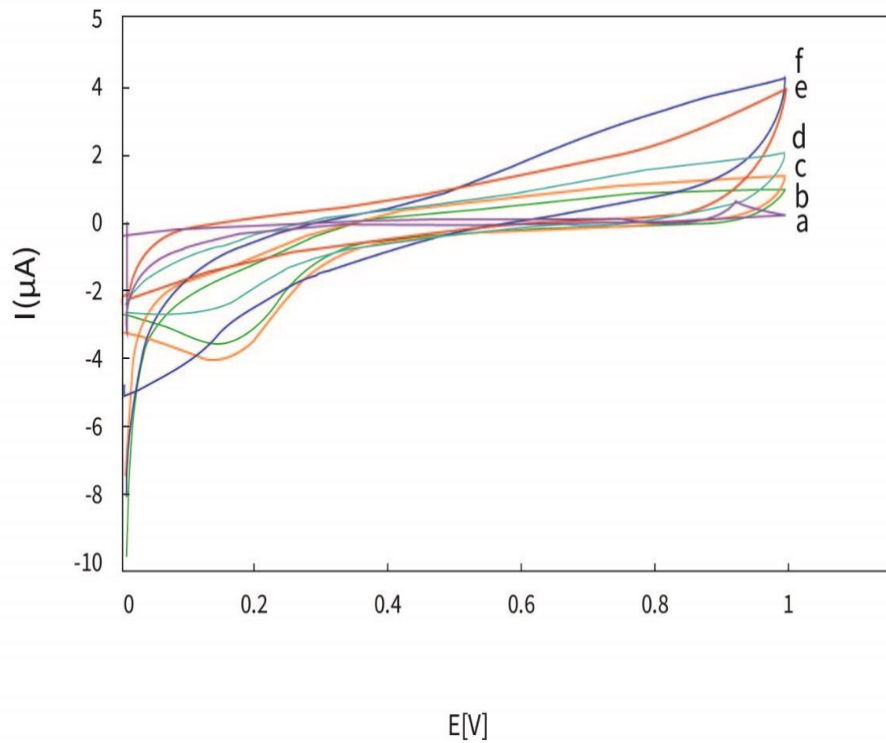
شکل شماره ۳. ولتاموگرام‌های ثبت شده از زیست حسگر مبتنی بر گلوتامات اکسیداز در غلظت‌های مختلف گلوتامات، غلظت (a) ۶۳ \mu\text{M} ، (b) ۱۲۵ \mu\text{M} ، (c) ۲۵۰ \mu\text{M} ، (d) ۵۰۰ \mu\text{M} ، (e) ۷۵۰ \mu\text{M} ، (f) ۱ mM، دما ۲۵ درجه سانتی گراد و pH ۷/۴
