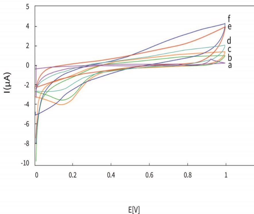
شکل شماره ۳. ولتاموگرام‌های ثبت شده از زیست حسگر مبتنی بر گلوکاتامات اکسیداز در غلظت‌های مختلف گلوکاتامات، غلظت (a) ۶۳ \mu\text{M} ، (b) ۱۲۵ \mu\text{M} ، (c) ۲۵۰ \mu\text{M} ، (d) ۵۰۰ \mu\text{M} ، (e) ۷۵۰ \mu\text{M} ، (f) ۱ mM، دما ۲۵ درجه سانتی‌گراد و pH ۷/۴
