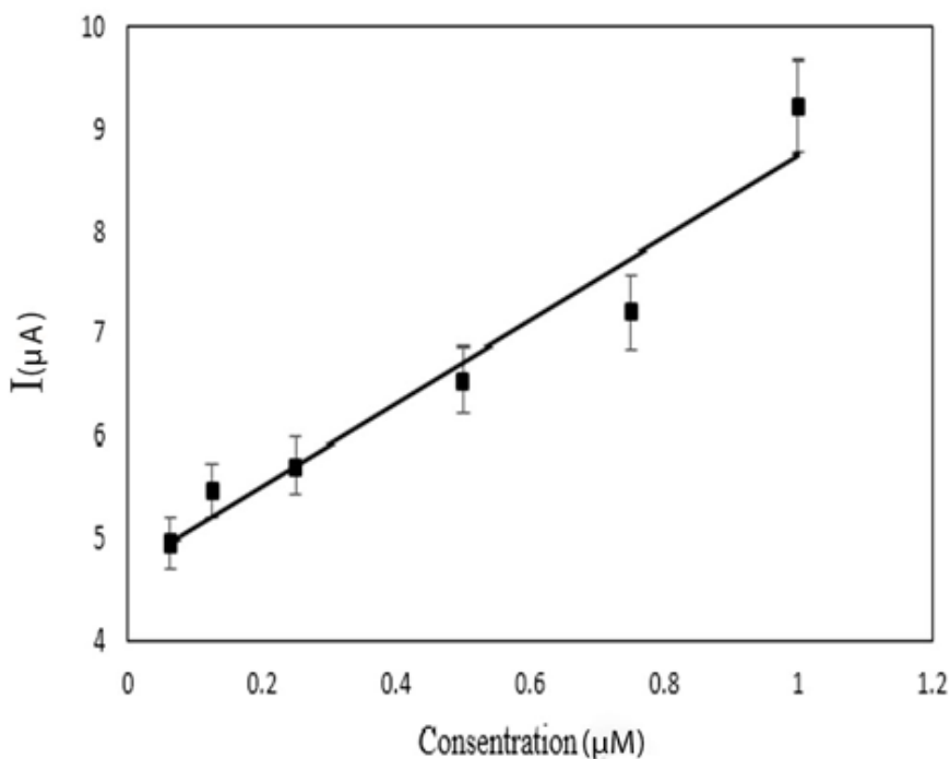
شکل شماره ۴. منحنی کالیبراسیون زیست حسگر مبتنی بر گلوکاتامات اکسیداز در غلظت‌های مختلف گلوکاتامات اندازه‌گیری گلوکاتامات در نمونه‌ی مغزی: بررسی عملکرد زیست حسگر الکتروشیمیایی مبتنی بر آنزیم
