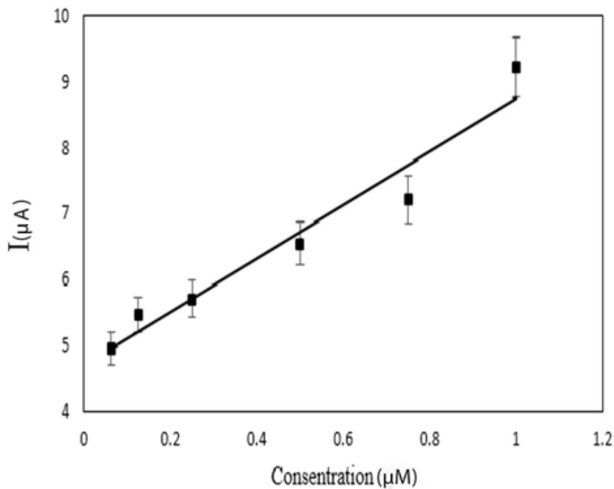
شکل شماره ۴. منحنی کالیبراسیون زیست حسگر مبتنی بر گلوتامات اکسیداز در غلظت‌های مختلف گلوتامات اندازه‌گیری گلوتامات در نمونه‌ی مغزی: بررسی عملکرد زیست حسگر الکتروشیمیایی مبتنی بر آنزیم
