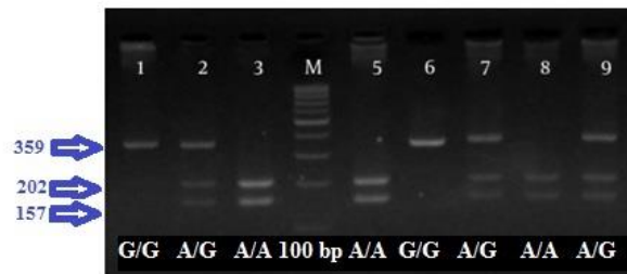
شکل شماره ۲. نماینده یک الکتروفورز ژل آگارز محصولات جزئی PCR از ژن CK-MM. چاهک‌های ۱ و ۶ نشان‌دهنده ژنوتیپ GG، چاهک‌های ۳، ۵ و ۸ نشان‌دهنده ژنوتیپ AA، چاهک‌های ۲، ۷ و ۹ نشان‌دهنده ژنوتیپ AG و M لدر (100 bp) است.
