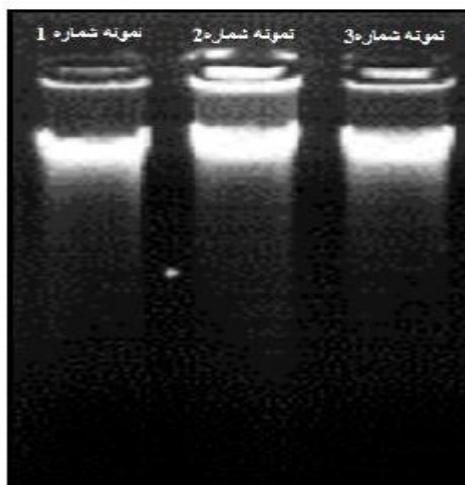
شکل شماره ۱. نتایج مربوط به استخراج DNA ژنومی از سلول‌های بزاقی انسانی روی ژل آگاروز ۱ درصد، تعداد ۳ نمونه (تیپیک)
