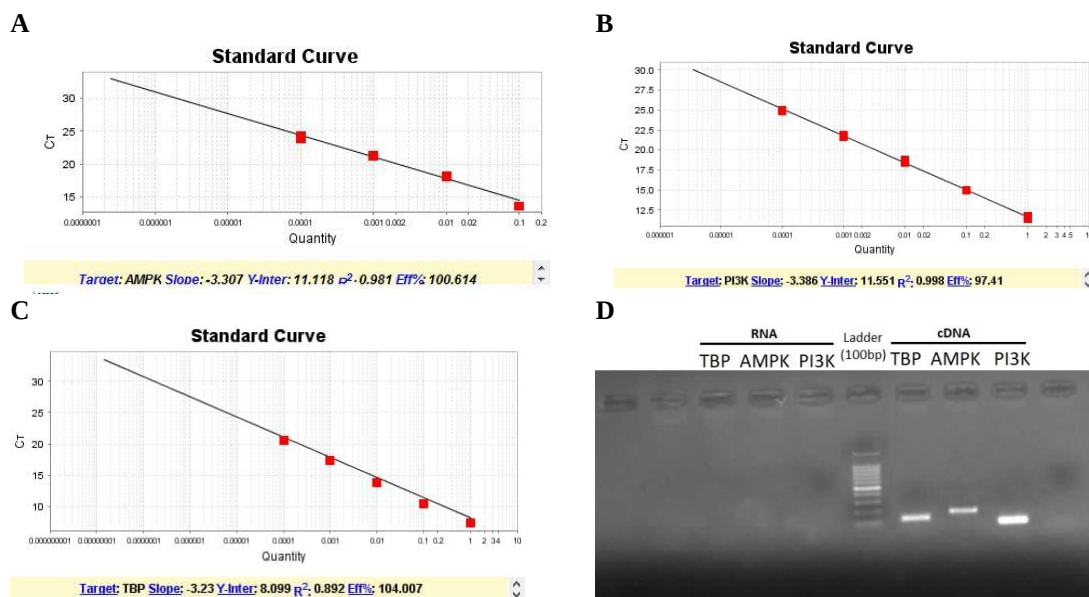
شکل شماره ۱. نمودارهای استاندارد و ژل الکتروفورز، منحنی استاندارد ژنهای AMPK (A)، PI3K (B) و ژن کنترل TBP (C). ژل الکتروفورز تکثیر PCR ژنهای TBP، AMPK و PI3K در حضور RNA استخراج شده و cDNA که نشان دهنده تکثیر نشدن ژن‌ها در حضور RNA استخراج شده (وجود نداشتن DNA ژنومی در نمونه استخراج RNA) و تکثیر ژن‌ها در نمونه cDNA است (D).
