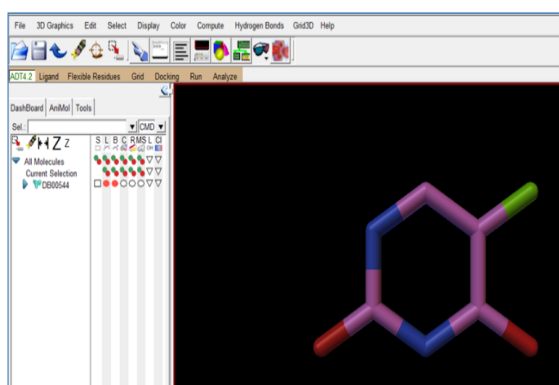
شکل شماره ۲. نمایش داروی فلوروآوراسیل با فرمت pdb در محیط نرم افزار داکینگ
