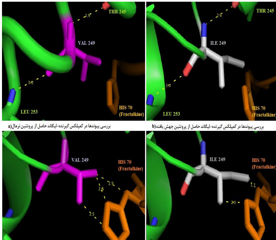
c) بررسی پیوند بین گیرنده و لیگاند در حالت نرمال
