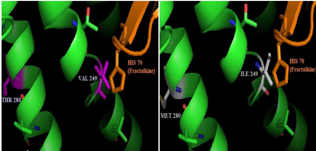
a) داکینگ مولکولی حاصل از پروتئین نرمال
