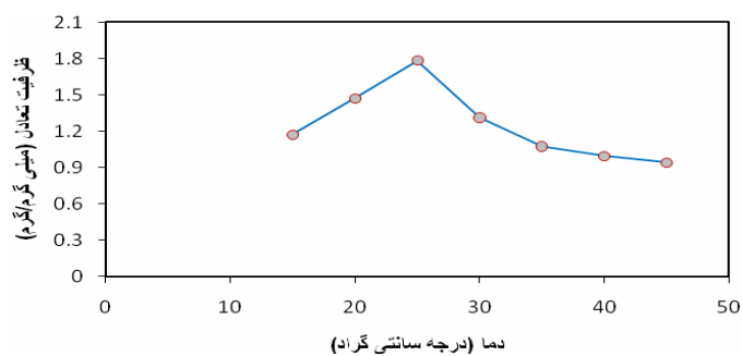
نمودار شماره ۲. اثر دماهای مختلف بر میزان جذب فلز مس در ساکارومیسس کارلبرژنزیس
