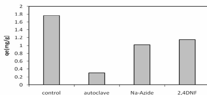
نمودار شماره ۶. مقایسه میزان جذب مس توسط ساکارومیسیس کارلبرژنزیس در حالت های فعال و غیرفعال از نظر متابولیسی
