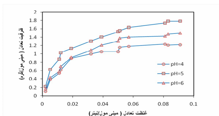
نمودار شماره ۴. اثر ایزوترم بر روی میزان جذب فلز مس توسط ساکارومیسس کارلبرژنزیس
