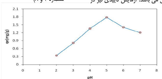
نمودار شماره ۱. اثر pH های مختلف بر میزان جذب مس توسط ساکارومیسس کارلبرنیزس
