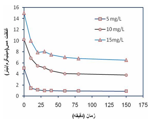
نمودار شماره ۳. اثر زمان بر روی میزان جذب فلز مس توسط ساکارومیسس کارلبرژنزیس
