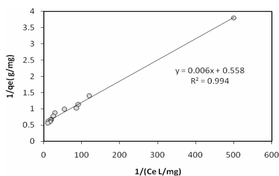
نمودار شماره ۵. ایزوترم بر روی میزان جذب فلز مس توسط ساکارومیسیس کارلبرژنزیس بر اساس مدل لانگمویر
