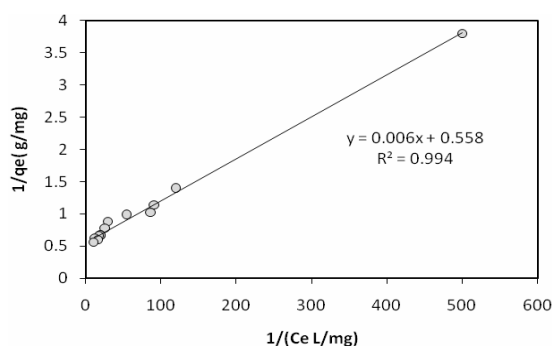
نمودار شماره ۵. ایزوترم بر روی میزان جذب فلز مس توسط ساکارومیسس کارلزبرژنزیس بر اساس مدل لانگمویر
