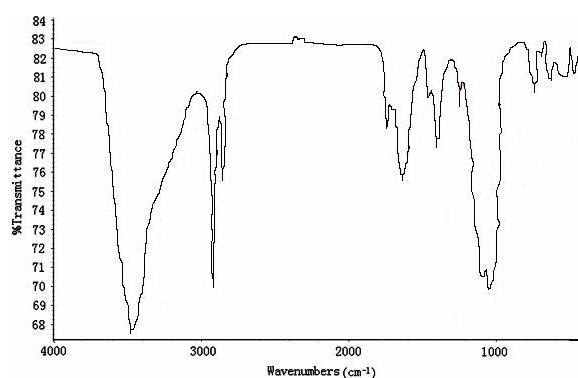
نمودار شماره ۷. تعیین گروه های شیمیایی سطح مخمر (بیک های منحنی) به وسیله FT-IR قبل اتصال فلز
