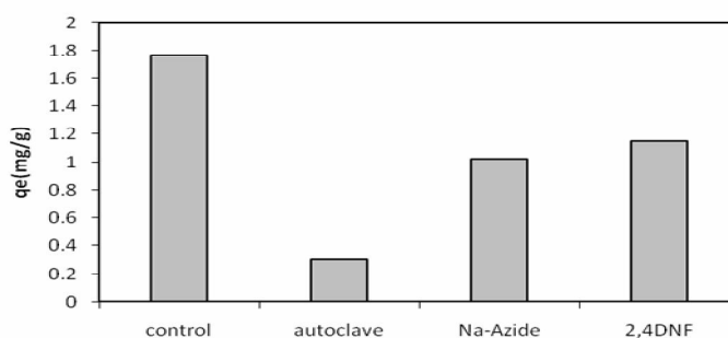
نمودار شماره ۶. مقایسه میزان جذب مس توسط ساکارومیسس کارلزبرژنزیس در حالت های فعال و غیرفعال از نظر متابولیسی
