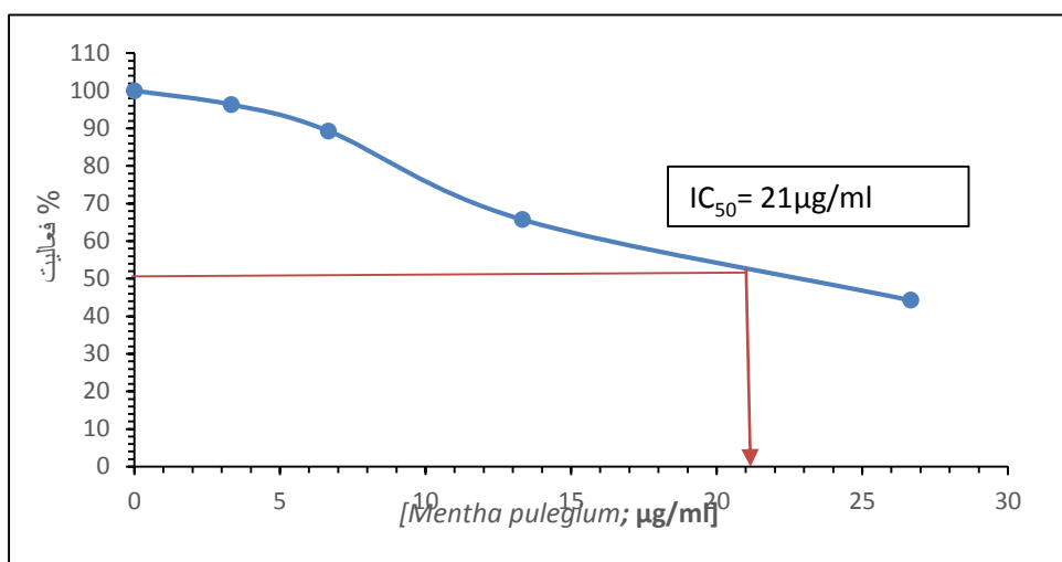
شکل شماره ۹. تغییرات باقیمانده فعالیت آنزیم استیل کولین استراز مغز گاو به ازای مقادیر مختلف از عصاره کونکوته. (فلش مقدار IC_{50} را نشان می دهد)
