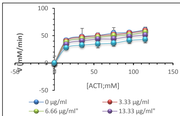
شکل شماره ۶. تغییرات سرعت واکنش کاتالیز شده با استیل کولین استراز در مجاورت غلظت های مختلف عصاره کوتکوته نمودار میکائلیس-منتن). (تمام اندازه گیری ها سه بار تکرار شد و مقادیر نشان داده شده انحراف معیار \pm مقدار میانگین می باشد).
