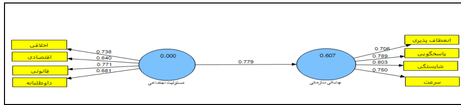
نمودار شماره ۲. مدل فرضیه اصلی تحقیق در حالت تخمین استاندارد
