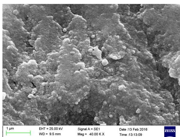
شکل شماره ۲. عکس میکروسکوپی الکترونی روبشی از نانوذرات نقره بیوستتز شده به روش زیستی
