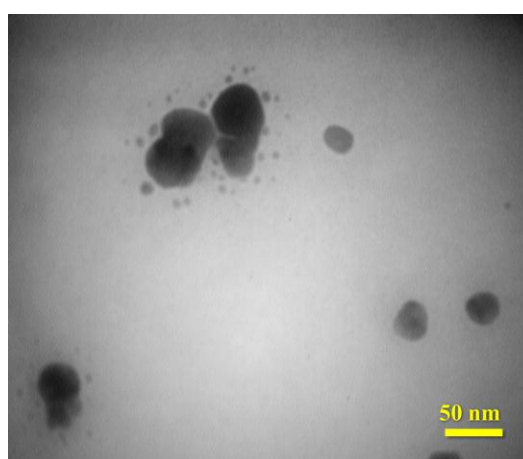
شکل شماره ۳. عکس میکروسکوپی الکترونی گذاره از نانوذرات نقره بیوستتز شده با جلبک قرمز L. caspica
