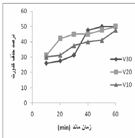
نمودار ۱۰. راندمان فرایند الکتروکواگولاسیون در حذف کلرورت
