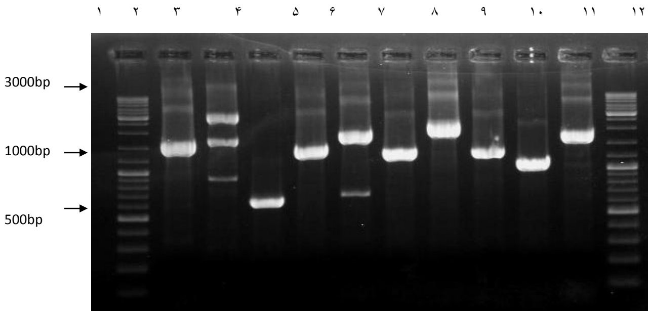
شکل شماره ۲. محصولات PCR پرایمرهای اختصاصی ژن های ناحیه Cag-PAI سویه هلیکوباکتری پیلوری ستون ۱ و ۱۲ Gene Ruler DNA Ladder Mix (Thermo Scientific)، ستون ۲ cagδ-cagδ (Wild (intact): ۱۰۹۲ bp)، ستون ۳ cagα-cagY (۱۸۱۸ bp)، ستون ۴ cagδ-cagγ (۱۴۱۷ bp)، ستون ۵ cagp-cagM (۶۰۱ bp)، ستون ۶ cagX-cagW (۱۳۰۶ bp)، ستون ۷ cagW-cagT (۲۲۸ bp)، ستون ۸ cagL-cagH (۱۳۲۹ bp)، ستون ۹ cagE-cagC (۱۰۸۳ bp)، ستون ۱۰ cagC-cagA (۱۹۱۷ bp)
