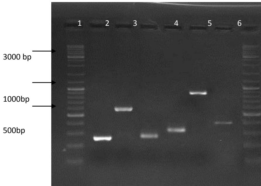
شکل شماره ۱. محصولات PCR ژن های vacA , cagA , iceA , babA . ستون ۱ و ۸ Gene Ruler DNA Ladder Mix (Thermo Scientific)، ستون ۲ ژن babA2 (۲۷۱ bp)، ستون ۳ ژن vacm1 (۵۶۷ bp)، ستون ۴ ژن vacs1 (۲۵۹ bp)، ستون ۵ ژن vacs2 (۲۸۶ bp)، ستون ۶ ژن iceA1 (۹۰۰ bp)، ستون ۷ ژن cagA (۴۰۰ bp)
