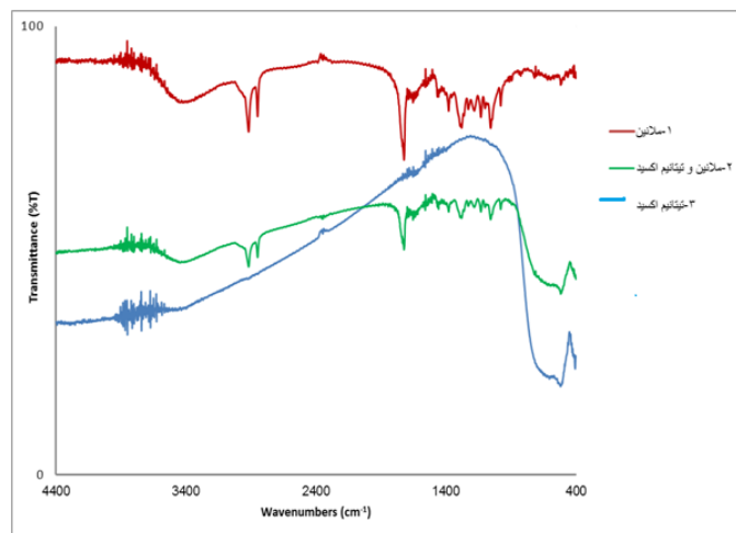
نمودار شماره ۱۰. FT-IR ۱-ملانین، ۲-ملانین-تیتانیوم اکسید، ۳-تیتانیوم اکسید
