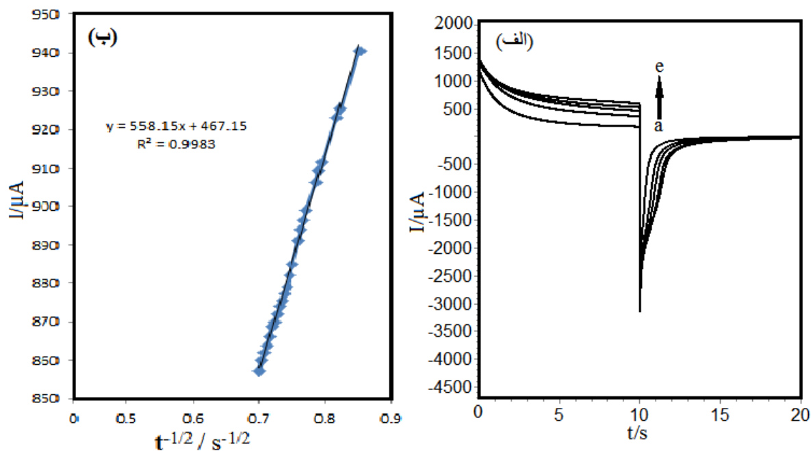
شکل (4) (الف) کروماتو آمپرو گرام به دست آمده در سطح Ni/NiZ/CPE در (a) غیاب (b) 1 \times 10^{-3} \text{ M} (c) 2/5 \times 10^{-3} \text{ M} (d) 1 \times 10^{-3} \text{ M} (e) 1/5 \times 10^{-3} \text{ M} از آموکسی سیلین در محلول 0/1 مولار سدیم هیدروکسید (ب) نمودار تغییرات I_C/I_L بر حسب t^{1/2} به دست آمده از کروماتو آمپرو گرام های (a) و (e) از قسمت (الف)
