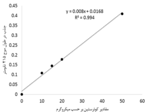
شکل شماره ۱. منحنی استاندارد؛ گالیک اسید جهت اندازه‌گیری مقادیر فنل (راست)، کوئرتستین جهت اندازه‌گیری مقادیر فلاونوئید (چپ)
