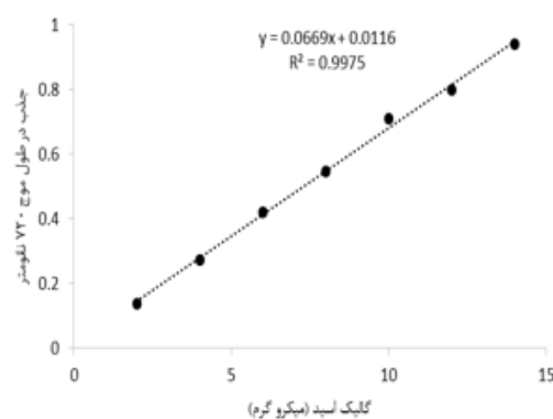
شکل شماره ۱. منحنی استاندارد؛ گالیک اسید جهت اندازه‌گیری مقادیر فنل (راست)، کوئرتستین جهت اندازه‌گیری مقادیر فلاونوئید (چپ)
