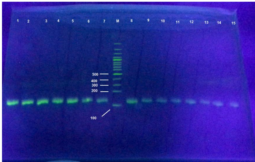
شکل ۱. الکتروفورز محصول PCR ژن 16srRNA برای تأیید جدایه های کلبرسیلا پنومونیه . ستون ۱: کنترل مثبت کلبرسیلا پنومونیه ، ستون های ۱۵-۲: نمونه های مثبت کلبرسیلا پنومونیه ، ستون M: مارکر ۱۰۰ جفت بازی.
