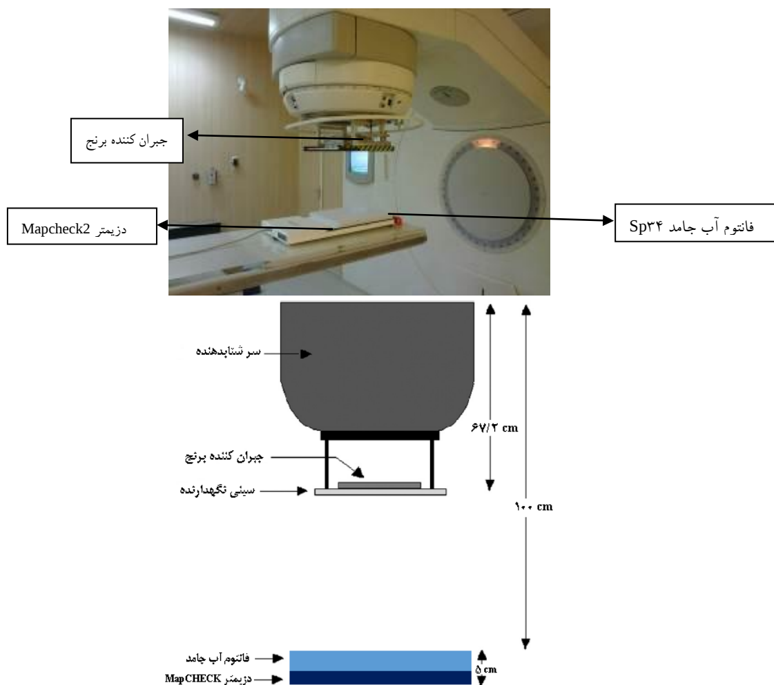
شکل شماره ۱. نحوه قرارگیری جبران کننده، فانتوم و دزیمر. بالایی: یک تصویر واقعی، و پایینی: یک تصویر شماتیک.
