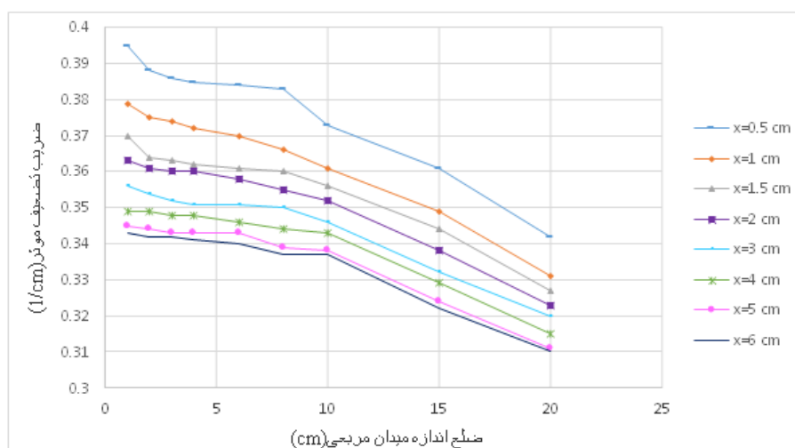
شکل شماره ۳. تغییرات ضریب تضعیف موثر بر حسب اندازه میدان
