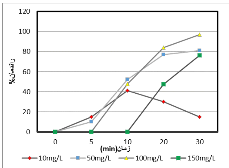
نمودار ۳: تأثیر غلظت‌های مختلف ۴- کلرو فنی بر کارایی سیستم O_3/H_2O_2 ([H_2O_2]=0.001 M, O_3=0.09 g/hr) pH=9
