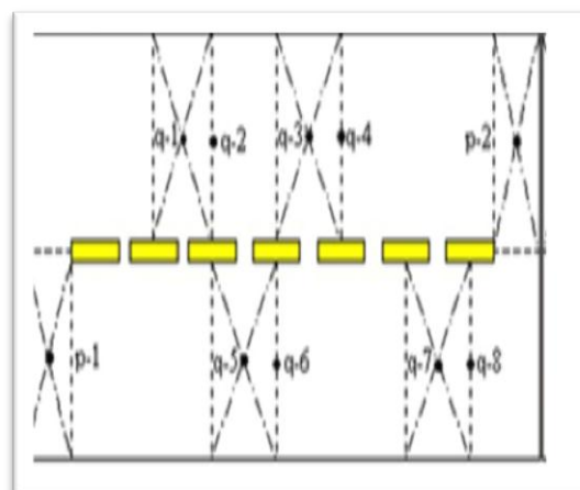
شکل شماره ۱. الگوی سوم در اندازه گیری روشنایی عمومی داخلی.
