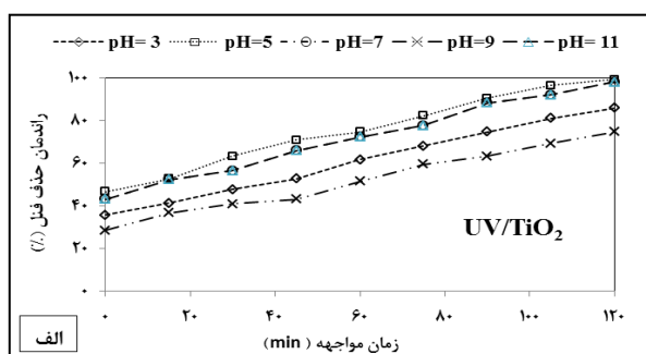
شکل شماره ۳. تاثیر \text{pH} بر کارایی حذف فنل (الف) ( \text{Phenol}=15 \text{ mg/L} , \text{Cd}=5 \text{ mg/L} , دوز \text{TiO}_2=1 \text{ g/L} و \text{min}=120 زمان مواجهه) و کادمیوم (ب) ( \text{Phenol}=5 \text{ mg/L} , \text{Cd}=15 \text{ mg/L} ) توسط فرآیند \text{UV/TiO}_2 در مدت زمان واکنش مشخص
