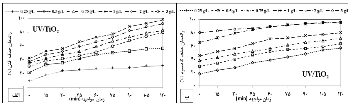
شکل شماره ۲. تاثیر مقدار نانوذرات بر کارایی حذف فنل (الف) ( Phenol=15\text{ mg/L} , Cd=5\text{ mg/L} , pH=7 و 120\text{ min} زمان مواجهه) و کادمیوم (ب) ( Phenol=5\text{ mg/L} , Cd=15\text{ mg/L} ) توسط فرآیند UV/TiO_2 در مدت زمان واکنش مشخص
