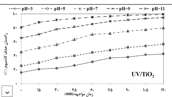
شکل شماره ۳. تاثیر \text{pH} بر کارایی حذف فنل (الف) ( \text{Phenol}=15 \text{ mg/L} , \text{Cd}=5 \text{ mg/L} , دوز \text{TiO}_2=1 \text{ g/L} و \text{min}=120 زمان مواجهه) و کادمیوم (ب) ( \text{Phenol}=5 \text{ mg/L} , \text{Cd}=15 \text{ mg/L} ) توسط فرآیند \text{UV/TiO}_2 در مدت زمان واکنش مشخص
