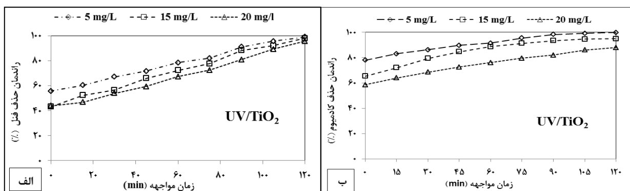
شکل شماره ۴. تاثیر غلظت اولیه بر کارایی حذف فنل (الف) ( \text{pH}=7 , \text{Cd}=5 \text{ mg/L} , دوز \text{TiO}_2=1 \text{ g/L} و \text{time}=120 \text{ min} ) و کادمیوم (ب) ( \text{pH}=7 , \text{phenol}=5 \text{ mg/L} , دوز \text{TiO}_2=2 \text{ g/L} ) بر کارایی حذف فنل توسط فرآیند \text{UV/TiO}_2 در مدت زمان واکنش مشخص
