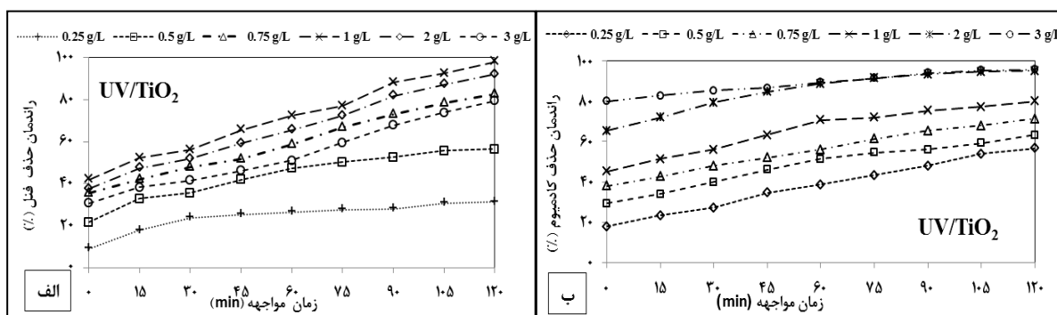
شکل شماره ۲. تاثیر مقدار نانوذرات بر کارایی حذف فنل (الف) ( pH=7 , Cd=5\text{ mg/L} , Phenol=15\text{ mg/L} ) و زمان 120\text{ min} و کادمیوم (ب) ( Phenol=5\text{ mg/L} , Cd=15\text{ mg/L} ) توسط فرآیند UV/TiO_2 در مدت زمان واکنش مشخص
