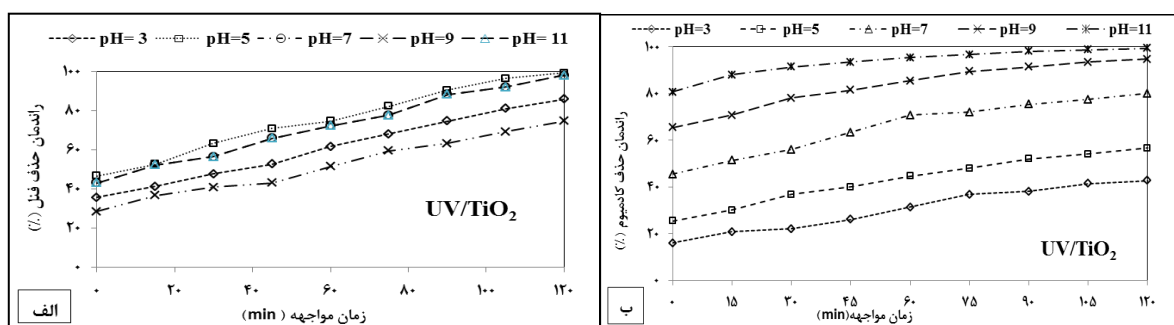
شکل شماره ۳. تاثیر \text{pH} بر کارایی حذف فنل (الف) ( \text{Phenol}=15 \text{ mg/L} , \text{Cd}=5 \text{ mg/L} , دوز \text{TiO}_2=1 \text{ g/L} و \text{time}=120 \text{ min} ) و کادمیوم (ب) ( \text{Phenol}=5 \text{ mg/L} , \text{Cd}=15 \text{ mg/L} ) توسط فرآیند \text{UV/TiO}_2 در مدت زمان واکنش مشخص
