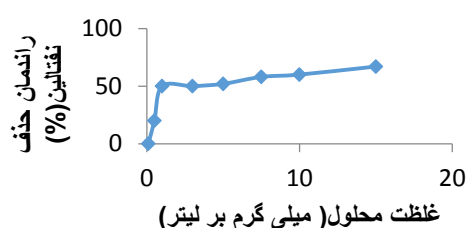
نمودار شماره ۳. بررسی تاثیر غلظت اولیه نفتالین بر کارایی حذف نفتالین از آب با نانولوله کربنی چند دیواره (دوز جاذب ۳/۰ گرم بر لیتر و زمان تماس ۹۰ دقیقه)
