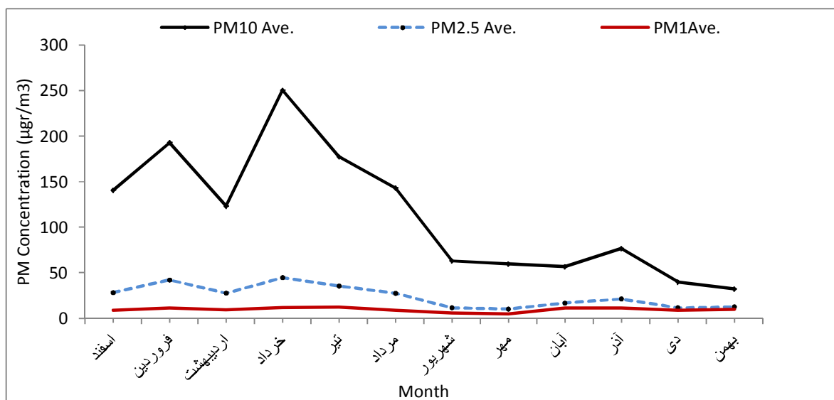
نمودار شماره ۳. روند تغییرات میانگین غلظت ماهیانه ذرات PM_{10} ، PM_{2.5} و PM_1 در دوره یک ساله (۱۳۹۱-۹۲) شهر ایلام
