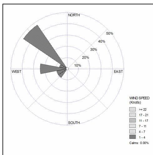
نمودار شماره ۱۰. گلباد جهت ورود طوفان های گرد و غبار به شهر ایلام در طول دوره نمونه برداری سال ۱۳۹۱-۹۲
