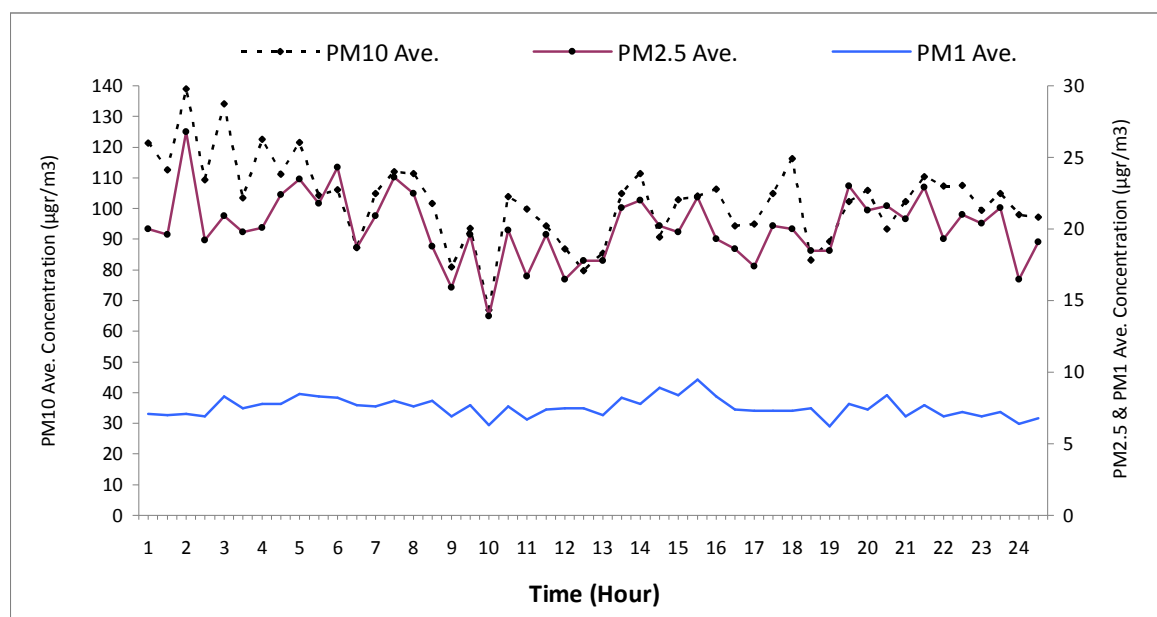
نمودار شماره ۴. روند تغییرات ساعتی میانگین غلظت PM_{10} ، PM_{2.5} و PM_1 در شبانه روز در طول دوره یک ساله (۱۳۹۱-۹۲) شهر ایلام
