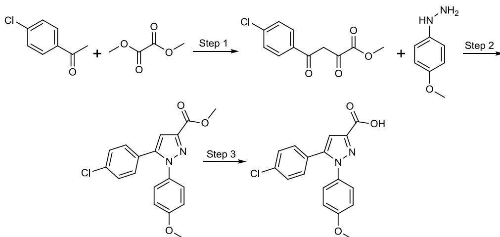
شکل شماره ۳. مراحل سنتز داروی شماره ۲
