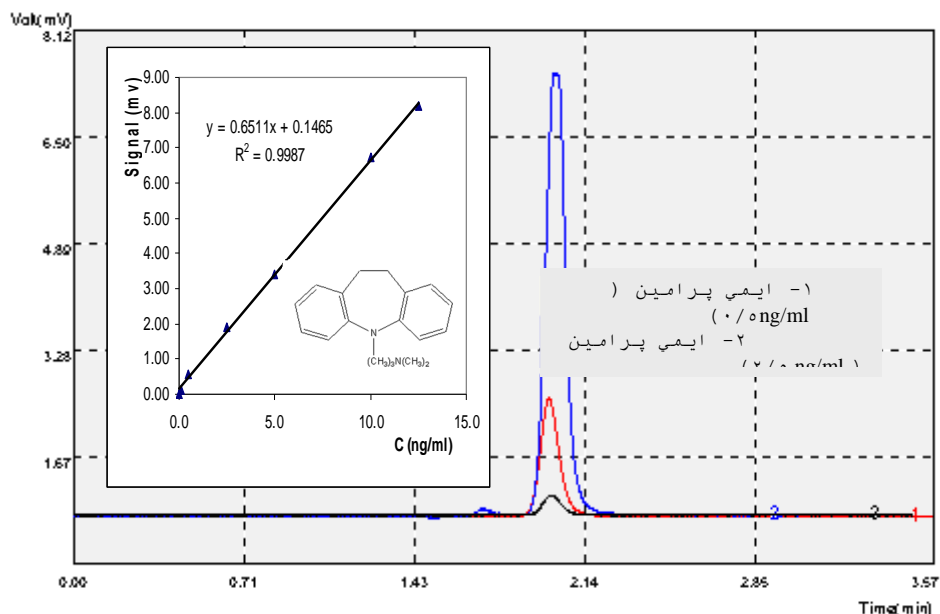
شکل 1. کروماتوگرام و منحنی کالیبراسیون ایمی پرامین مربوط به تعیین مقدار ماده مؤثره و میزان یکنواختی ایمی پرامین در قرص های 10 و 50 میلی گرمی (شرایط دستگاهی شامل ستون: (PRP-1 (4/1 × 150 mm ، 10 μm) در دمای +40°C ، فاز متحرک: استونیتریل: محلول بافر فسفات (62:38 در pH=4/0) با سرعت جریان 1/5 ml/min، طول موج تهییج: 250 نانومتر و طول موج نشر فلورسانس: 360 نانومتر)
