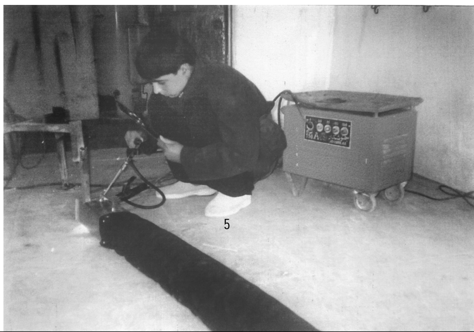
قرارگیری هود مکش هنگام کار بر روی قطعه L شکل
