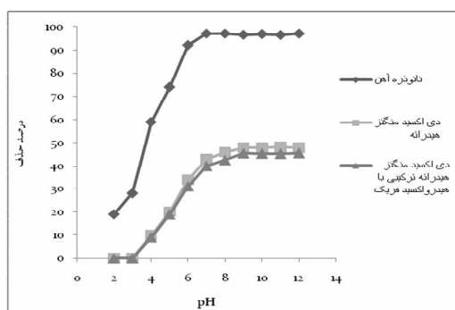
شکل شماره ۲. تأثیر pH در حذف یون کادمیوم با غلظت اولیه \text{mg/L} ۱۰ برای محلول سنتتیک توسط نانو ذرات آهن صفر ظرفیتی و ترکیبات منگنزی در زمان تماس ۶۰ دقیقه
