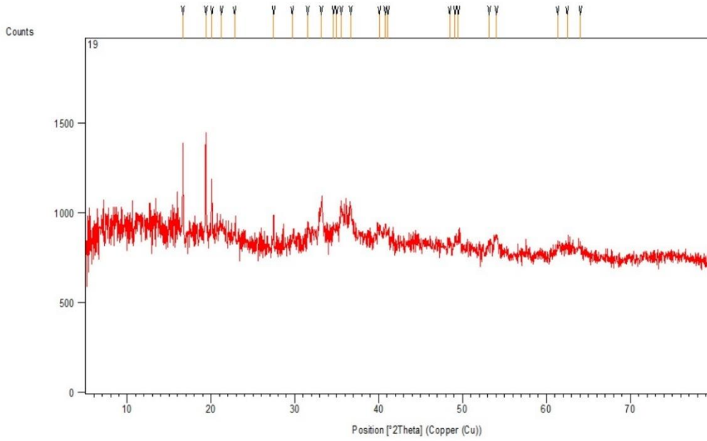
شكل شماره ۲. تجزيه و تحليل XRD نانوذرات Fe 3 O 4 @Glu-Coumarin
