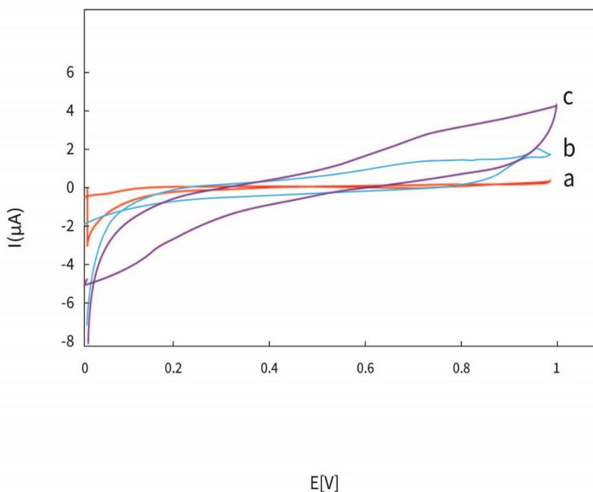
شکل شماره ۲. ولتاموگرام منحنی پایه (a)، ولتاموگرام زیست حسگر مبتنی بر گلوتامات اکسیداز در غلظت 250 \mu M H_2O_2 (b)، ولتاموگرام
