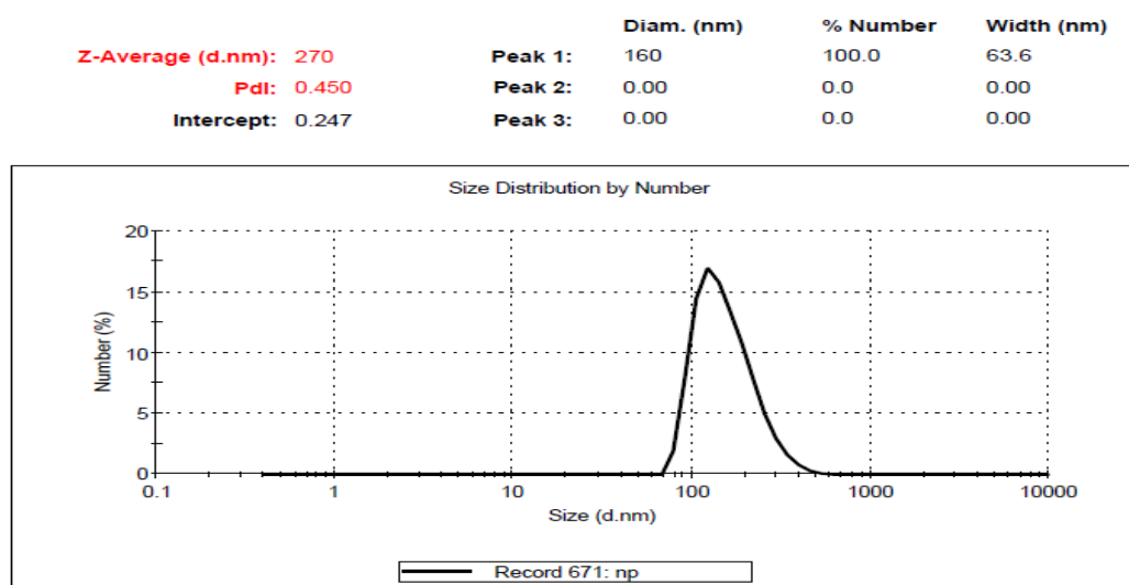
شکل شماره ۴. نمودار بررسی بازه توزیع اندازه نانوذرات تری‌متیل کایتوزان حاوی پروتئین BLF1-StxB در شرایط بهینه توسط دستگاه DLS
