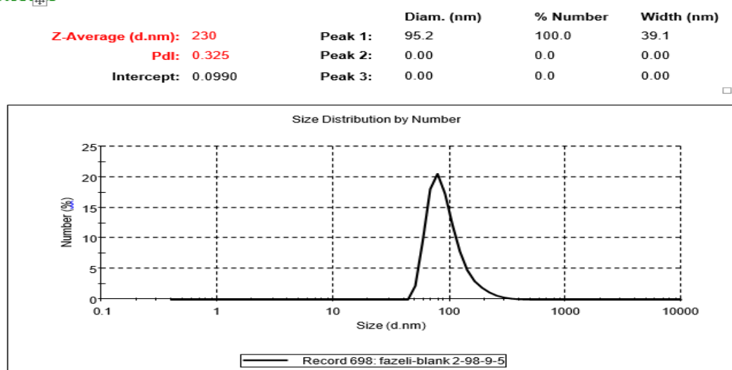
شکل شماره ۳. نمودار بررسی بازه توزیع اندازه نانوذرات تری‌متیل کایتوزان بدون پروتئین BLF1-StxB در شرایط بهینه توسط دستگاه DLS
