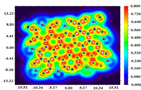
شکل شماره ۱۲. توپوگرافی دوبعدی جذب مولکول جنستین بر صفحه گرافن دپ شده با اتم های Ni در فاصله ۱/۱۸۰ (انگستریم)
