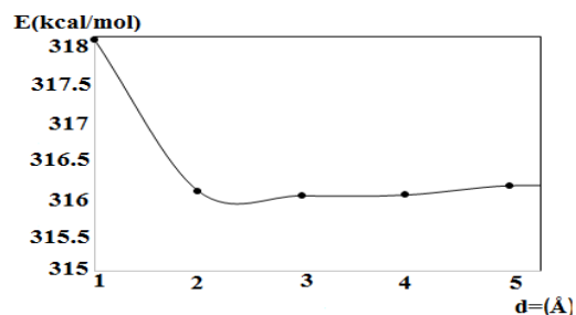
شکل شماره ۸. انرژی جذب مولکول دارویی جنستین و صفحه گرافن دوپ شده با اتم های Ni بر حسب فاصله (انگسترم)
