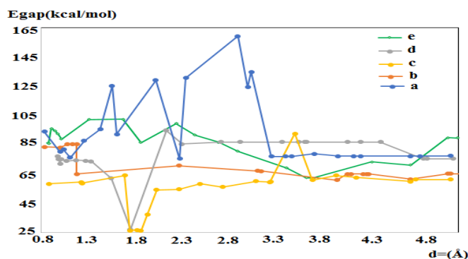
شکل شماره ۱۱. شکاف انرژی مولکول جنستین و صفحه گرافن دوپ شده با اتم‌های (a) G-Ge، (b) Ni-G-Ge، (c) Ti-G-Ge، (d) Se-G-Ge و (e) Cr-G-Ge
