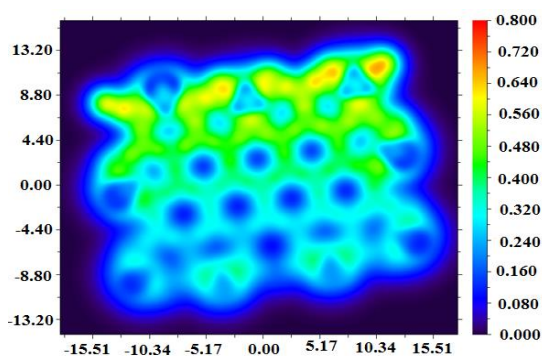
شکل شماره ۱۳. توپوگرافی دوبعدی جذب مولکول جنستین روی صفحه گرافن دپ شده با اتم های Ni در فاصله ۵/۱۱۲ (انگستریم)
