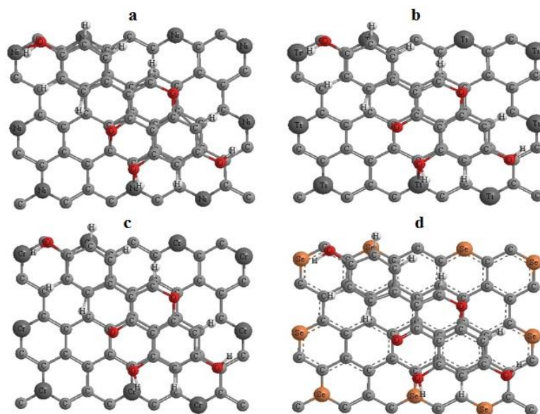
شکل شماره ۳. ساختار و موقعیت جذب مولکول داروی جنستین روی صفحه گرافن دپ شده با اتم‌های فلزی (a) Ni، (b) Ti، (c) Cr و (d) Se
