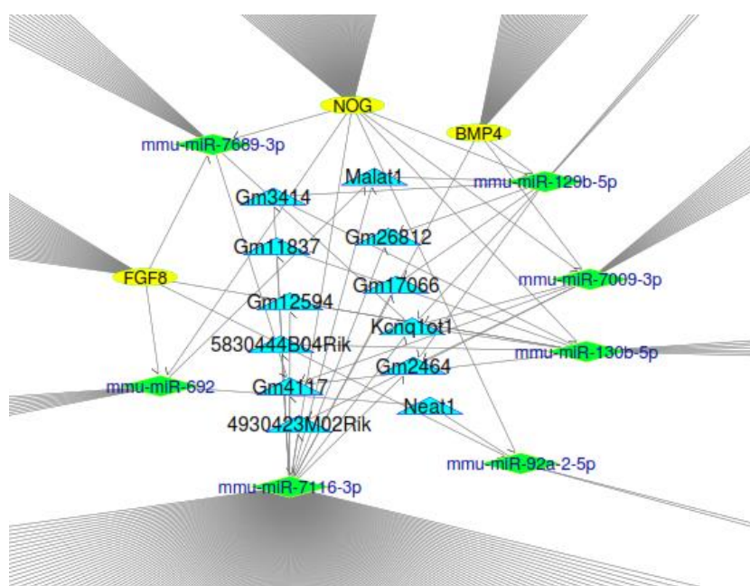
شکل شماره ۶. lncRNAهای مشترک میان miRNA. lncRNAهای هدف برای miRNAهای منتخب از سایت DIANATOOLS که امتیاز < ۰/۹۵ داشتند، استخراج و شبکه ژنی lncRNA-miRNA با استفاده از نرم افزار Cytoscape ترسیم شد. دایره های زرد رنگ نشان دهنده mRNA، لوزی های سبز رنگ miRNAهای مشترک و مثلث های آبی نشان دهنده lncRNAها است.
