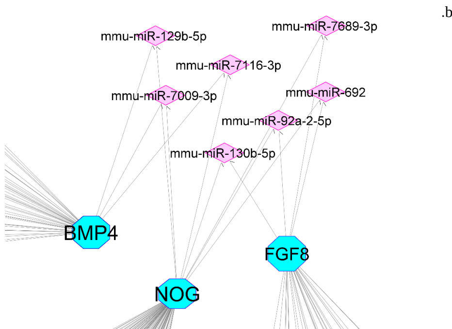
شکل شماره ۴: miRNAهای مشترک میان سه ژن BMP4, NOG و FGF8. پس از ترسیم شبکه ژنی mRNA-miRNA برای سه ژن BMP4, NOG و FGF8، miRNAهای مشترک انتخاب شدند. تصویر a شماتیک کلی است. تصویر b جزئی از شکل a است که برای نمایش جزئیات بیشتر آورده شده است. پنج ضلع‌های آبی، mRNA و لوزی‌های بنفش، miRNA هستند.
