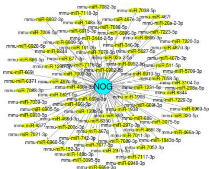
شکل شماره ۳: شبکه ژنی میان NOG و miRNAهای هدف آن. miRNAهای هدف ژن BMP4 از پایگاه داده‌ای MirWalk و TargetScan استخراج شد؛ سپس miRNAهای مشترک میان دو پایگاه داده‌ای انتخاب و با استفاده از نرم‌افزار Cytoscape، شبکه ژنی mRNA-miRNA برای ژن BMP4 رسم گردید.
