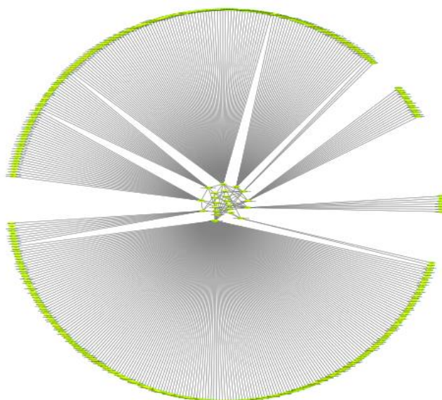
شکل شماره ۵. شبکه mRNA-miRNA-lncRNA. شبکه ژنی CeRNA (mRNA-miRNA-lncRNA) برای سه ژن پادشده BMP4، NOG و FGF8 با استفاده از نرم افزار Cytoscape رسم گردید.
