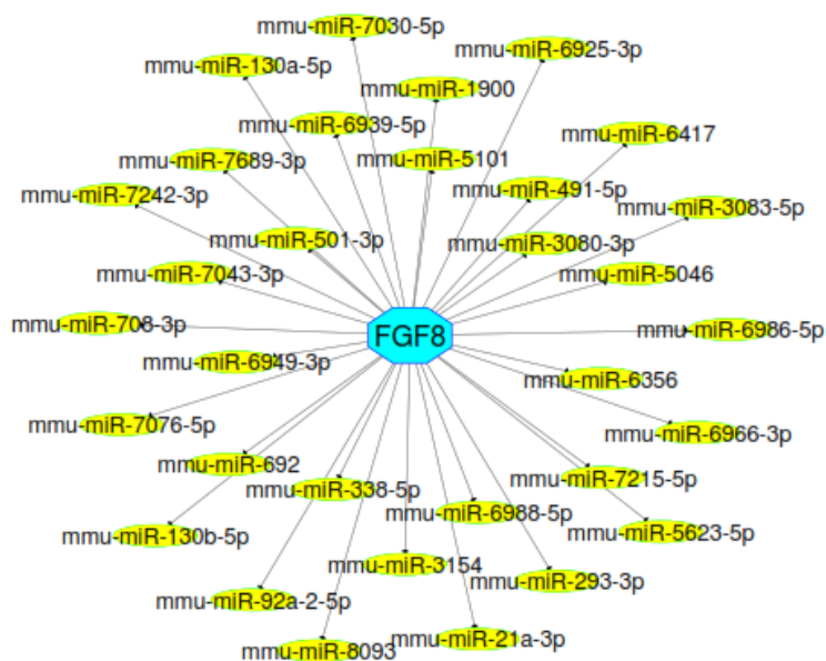
شکل شماره ۲. شبکه ژنی میان FGF8 و miRNAهای هدف آن. miRNAهای هدف ژن FGF8 از پایگاه داده‌ای MirWalk و TargetScan استخراج شد؛ سپس miRNAهای مشترک میان دو پایگاه داده‌ای انتخاب و با استفاده از نرم‌افزار Cytoscape، شبکه ژنی mRNA-miRNA برای ژن FGF8 رسم گردید.
