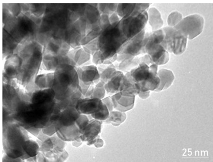
شکل شماره ۷. تصویر FETEM برای نانوذرات فریت روی سنتز شده
