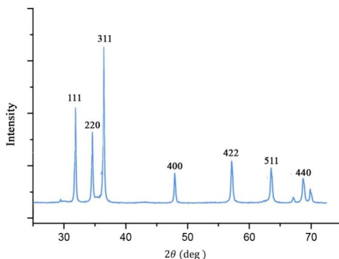
شکل شماره ۵. طیف سنجی پراش پرتوی ایکس (XRD) برای نانوذرات فریت روی ( \text{ZnFe}_2\text{O}_4 )
