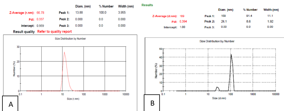
شکل ۲. نمودار بررسی بازه توزیع اندازه نانوذرات PEG-PLA حاوی پروتئین مخلوط PAD4+LFD1 (A) و بدون پروتئین (B) در شرایط بهینه توسط دستگاه DLS. منحنی‌های آزمون پراکندگی نور دینامیکی برحسب اندازه و توزیع (%).
