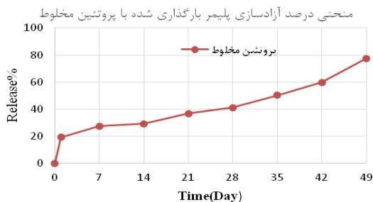
شکل ۱. نتایج درصد تجمعی رهایش پروتئین نوترکیب مخلوط از نانوذرات PEG-PLA در طول مدت ۴۹ روز. پس از گذشت ۴۹ روز، درصد رهایش پروتئین‌های مخلوط نوترکیب PAD4+LFD1 کپسوله‌شده در نانوذرات PLA-PEG حدود ۷۸ درصد تعیین گردید.
