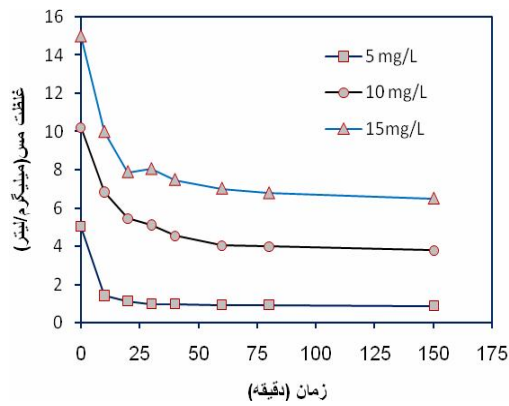
نمودار شماره ۳. اثر زمان بر روی میزان جذب فلز مس توسط ساکارومیسس کارلزبرژنزیس
