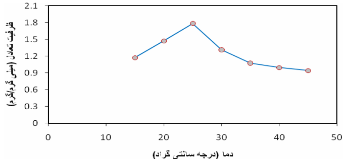
نمودار شماره ۲. اثر دماهای مختلف بر میزان جذب فلز مس در ساکارومیسس کارلزبرژنزیس
