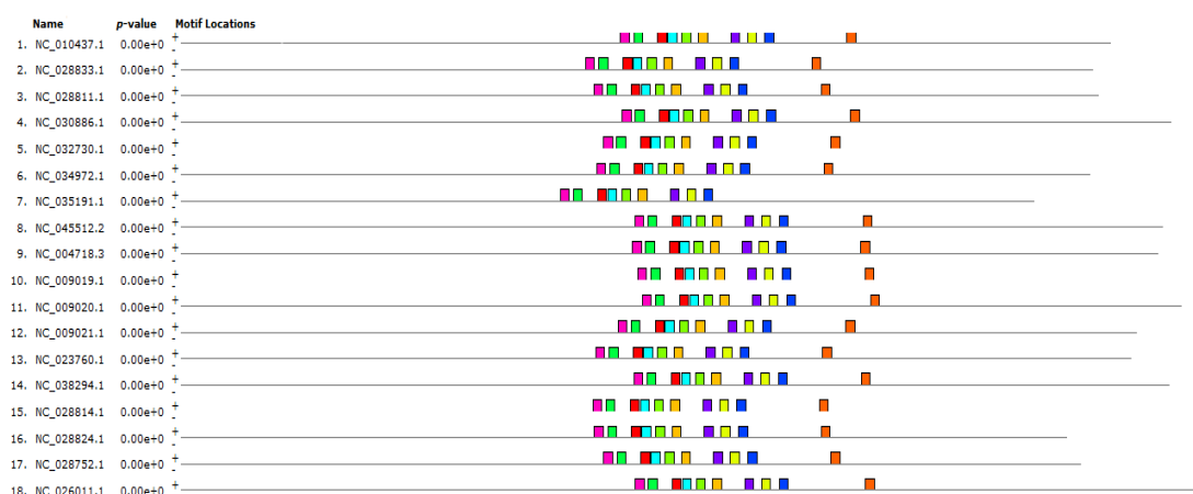
شکل شمارهٔ ۲. تعداد، نوع و موقعیت موتیف‌ها در ژنوم همهٔ ویروس‌های خانوادهٔ کرونا ارائه‌شده در سرچای NCBI
