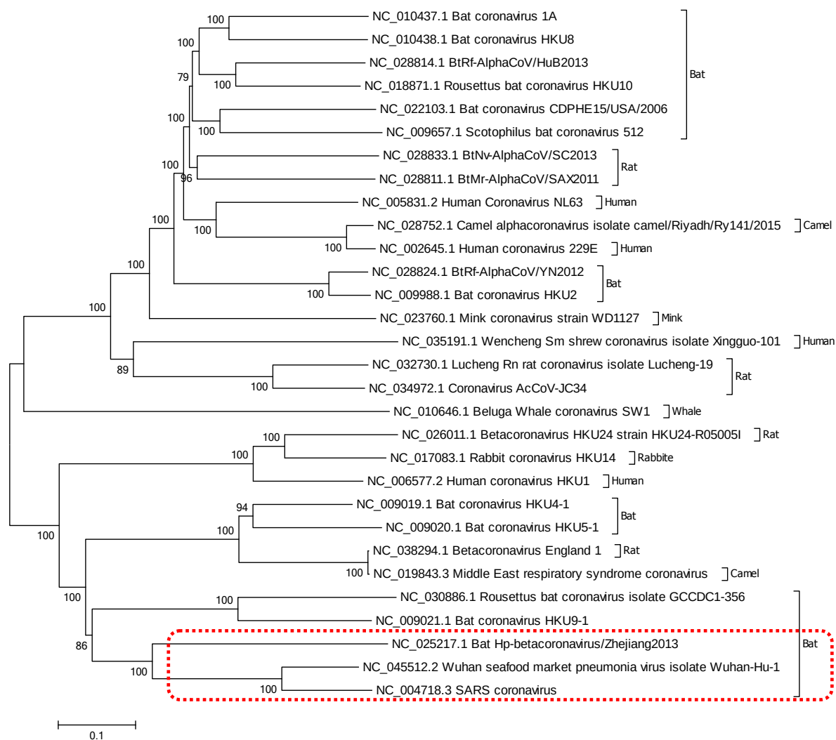
شکل شماره ۴. تجزیه خوشه‌ای حاصل از ژنوم ویروس‌های خانواده Coronaviridae بر اساس ماتریس فاصله نی و لی (Nei and Li) و روش NJ در نرم‌افزار Mega vol.6
