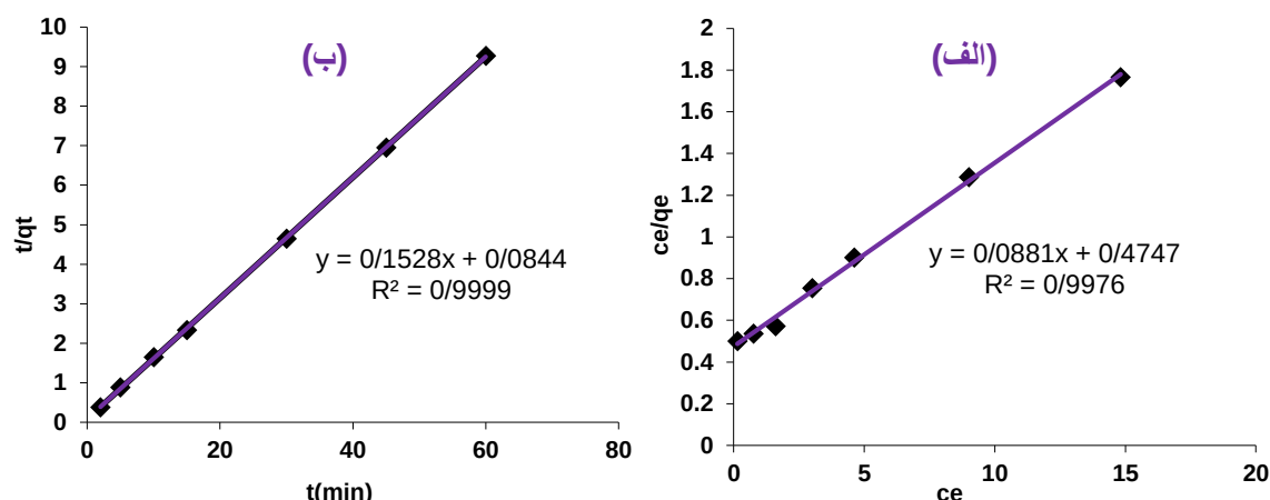
شکل شماره ۳. جذب آنتراسن توسط نانوجاذب سنتز شده بر اساس (الف) ایزوترم جذب لانگمویر (ب) ینتیک جذب شبه درجه دوم ( pH=7 ، دوز جاذب 0.7 گرم بر لیتر، زمان تماس 10 دقیقه، غلظت آنتراسن 20 میلی گرم بر لیتر)
