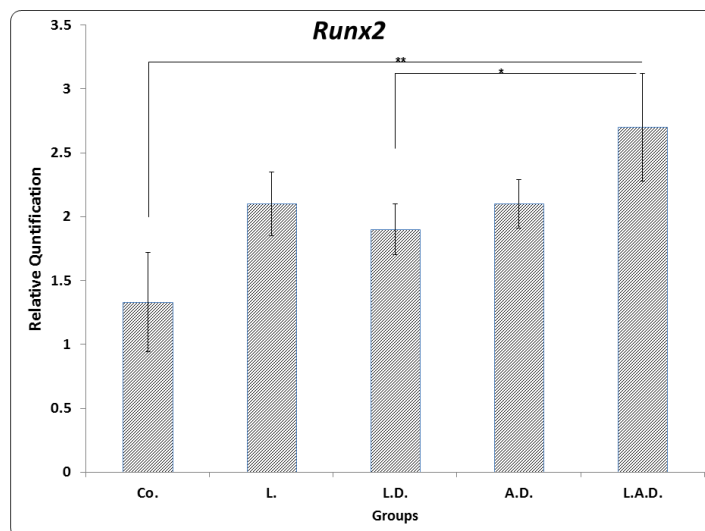
شکل شماره ۵. Mean±SEM برای بیان ژن Runx2 مقایسه بین گروه های مورد مطالعه به روش ANOVA و آزمون LSD (*P<0.05, **P<0.01)
