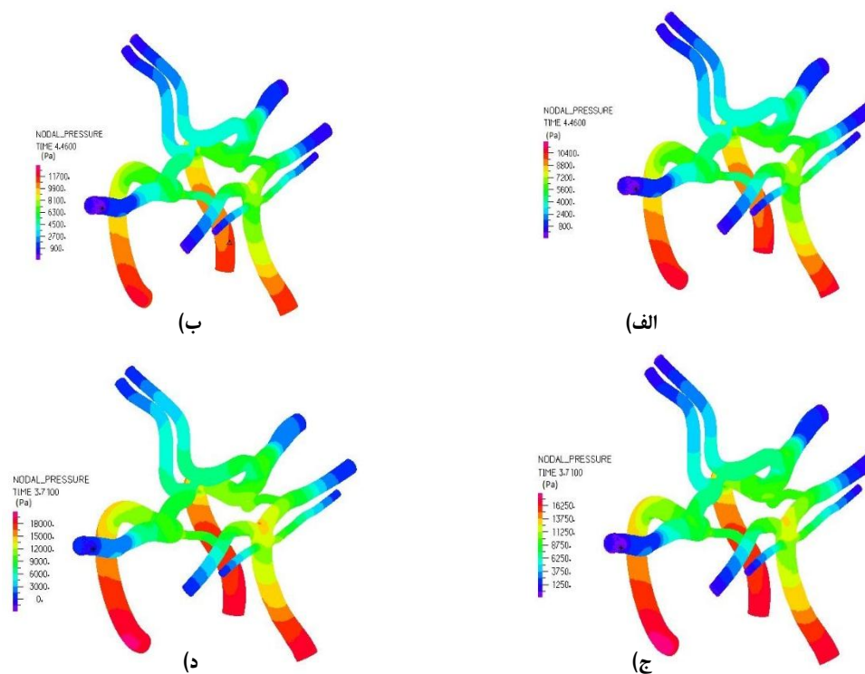
شکل شماره ۷. کانتور فشارخون در زمان الف) دیاستول در شرایط گرانش 1g ؛ ب) دیاستول در شرایط گرانش صفر؛ ج) سیستول در شرایط گرانش 1g ؛ د) سیستول در شرایط گرانش صفر
