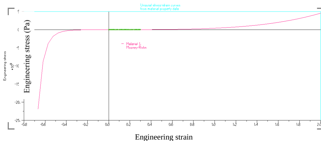
شکل شماره ۳. تنش بر حسب کرنش در مدل مونی ریولین، استفاده شده برای مدل هایپرالاستیک رگ. داده های حاصل از آزمایش تنش-کرنش یک محوره رگ با مدل مونی ریولین ۵ ثابت در آدینا برازش یافته است (۲۴)
