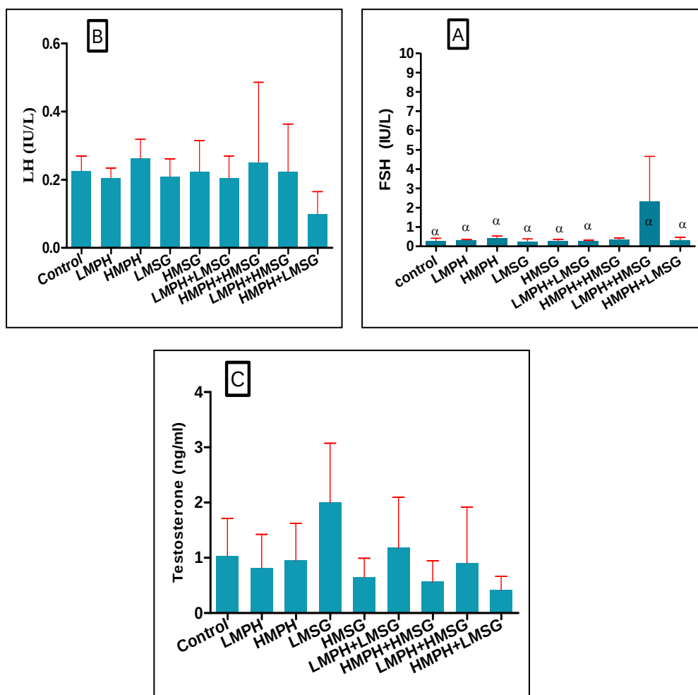
نمودار شماره ۱. سطوح سرمی گنادوتروپین های هیپوفیزی (A و B) و تستوسترون (C) در گروه های تحت مطالعه. داده ها به صورت \text{mean} \pm \text{SD} نشان داده شده است. ( \alpha ) اختلاف معنی دار ( P = 0.018 ) در مقایسه با گروه (Low MPH+ High MSG)
