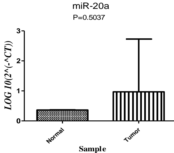
نمودار شماره ۴. مقایسه میزان بیان miR-20a در نمونه های توموری با نرمال
