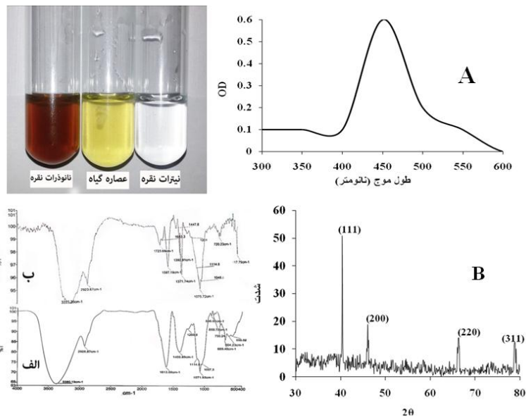
شکل شماره ۱- A: طیف UV/Visible مخلوط واکنش نیترات نقره ۱ میلی مولار و عصاره در غلظت ۱ میلی گرم بر میلی لیتر) از زرد به قهوه ای در دمای ۲۰ درجه سانتی گراد. B: تصویر پراش X-ray مربوط به نانوذرات نقره سنتز شده توسط عصاره بذر و طیف مادون قرمز (FTIR) عصاره الف: قبل از واکنش، ب: پس از واکنش
